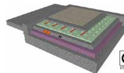
PLATEA-SOLAIO CONTROTERRA
